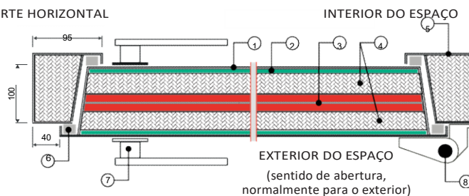
CORTE HORIZONTAL
