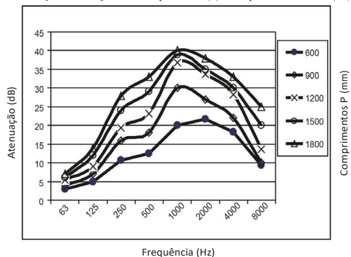
Ensaio LAIC 8-201/06 Atenuação em função do Comprimento (P) e Frequência do ruído (Hz)
